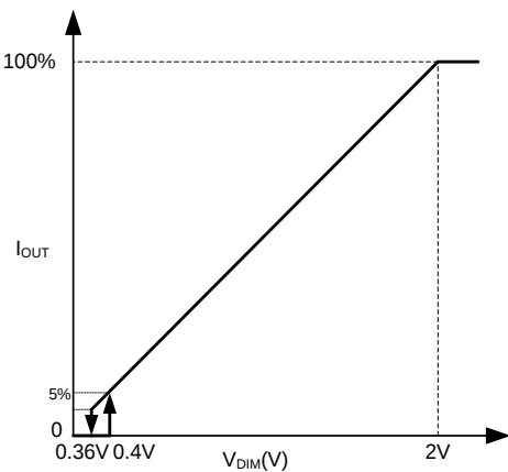
图 4 BP2308 模拟调光曲线
