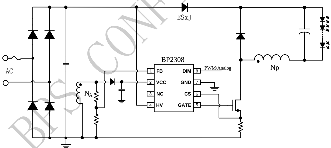
图 1 BP2308 典型应用图
