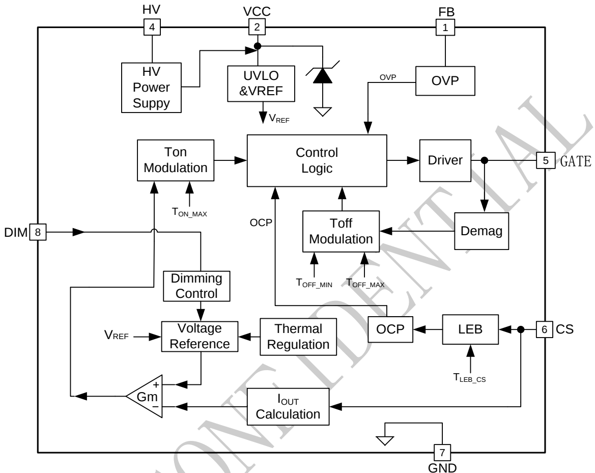
图 3 BP2308 内部框图
