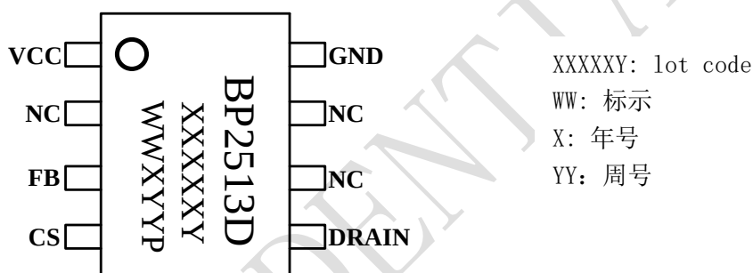
图 2 管脚封装图
