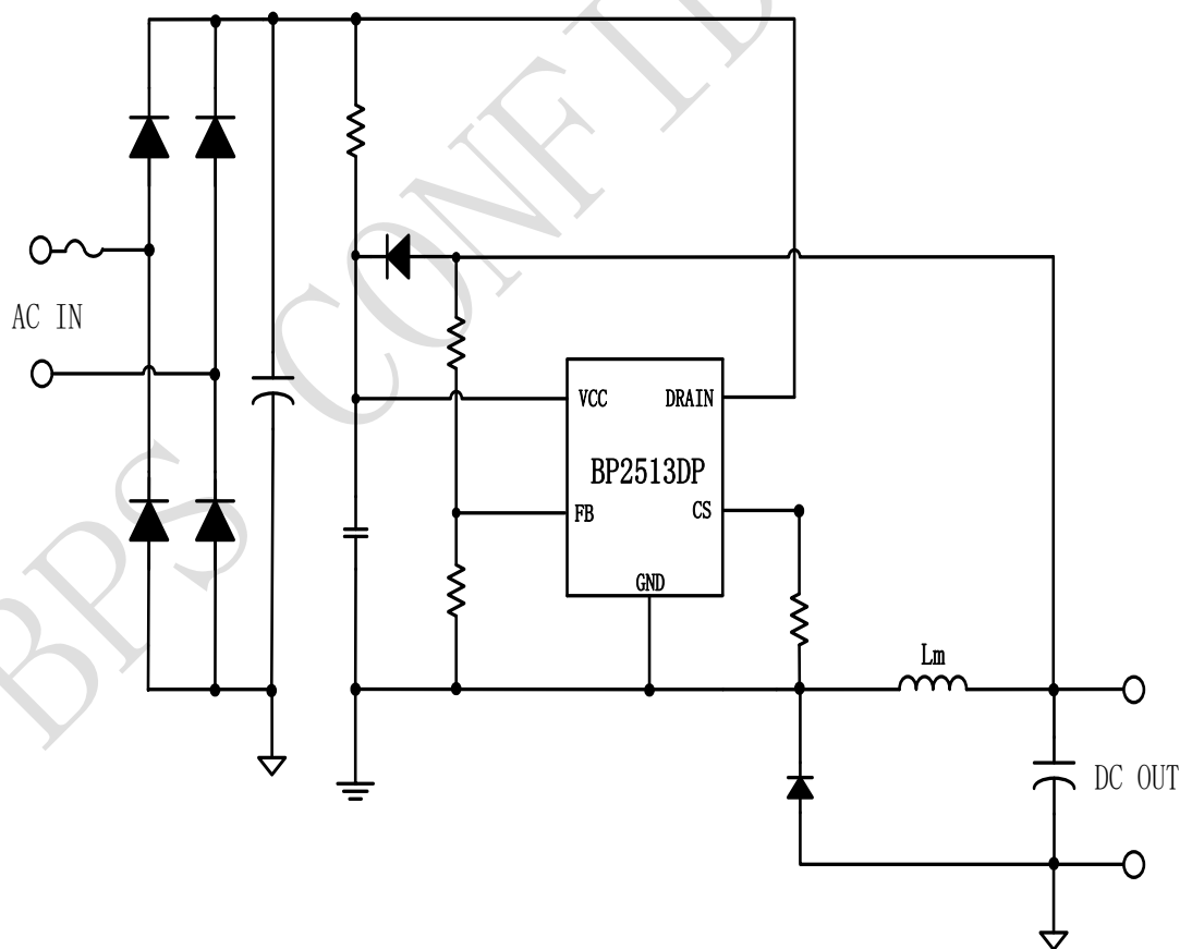
图 1 BP2513DP 典型应用图
