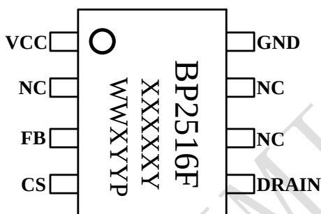
图 2 管脚封装图
