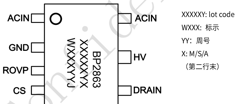
图 2 管脚封装图
