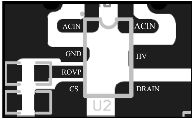
图 4 PCB 铺铜面积优化图
