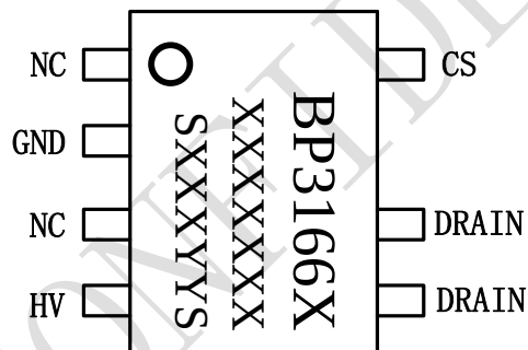
图 2 管脚封装图
