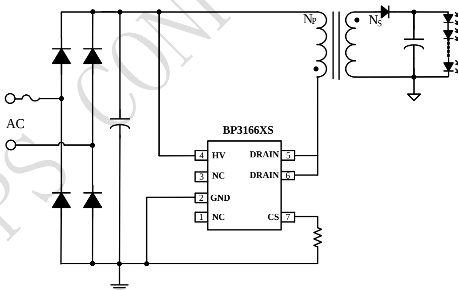
图 1 BP3166XS 典型应用图
