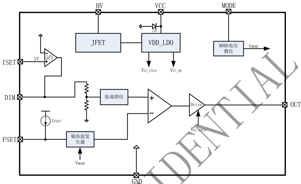
图 3 BP5001 内部框图
