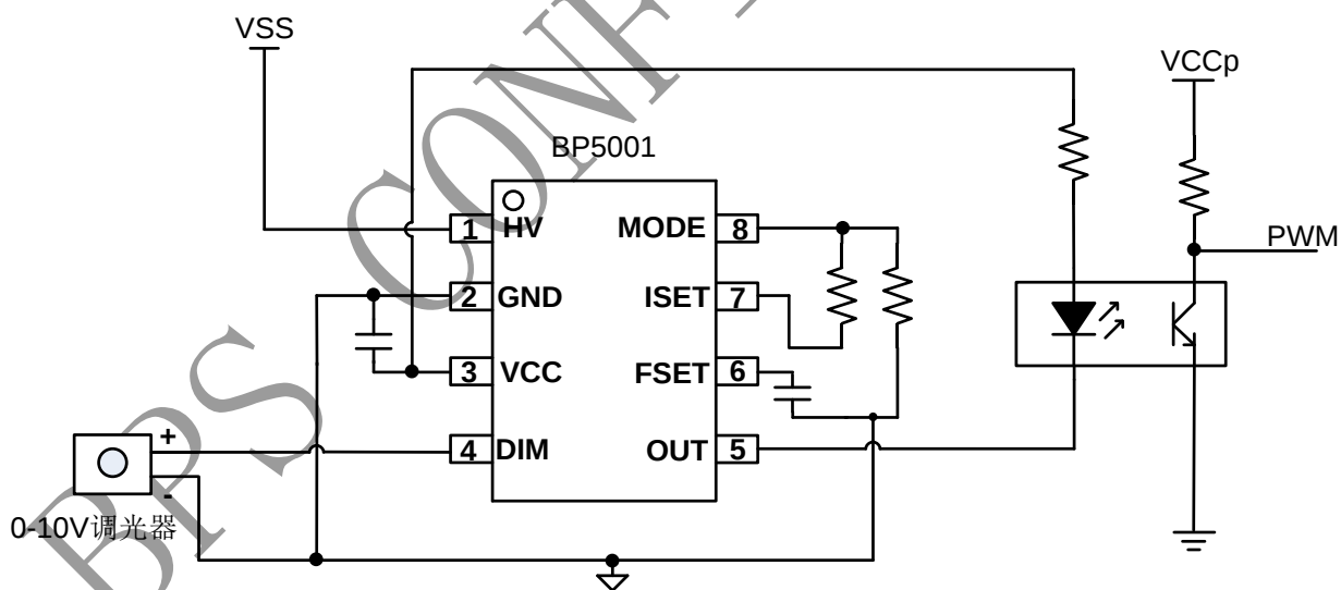
图 1 BP5001 典型应用图
